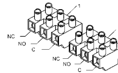
1 = Anschlussklemme Schalter A / Terminal block A switch / bornier microrupteur A 2 = Anschlussklemme Schalter B / Terminal block switch B / bornier microrupteur B
